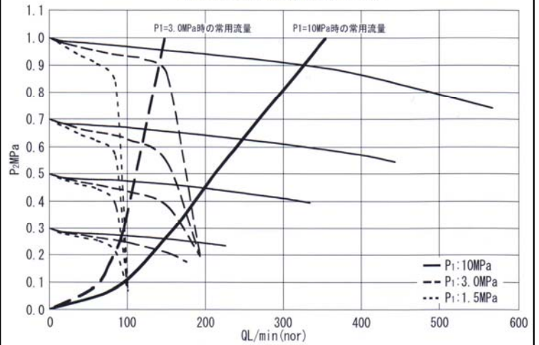
CMH-B506/B510/B515流量特性(N2ガス)
