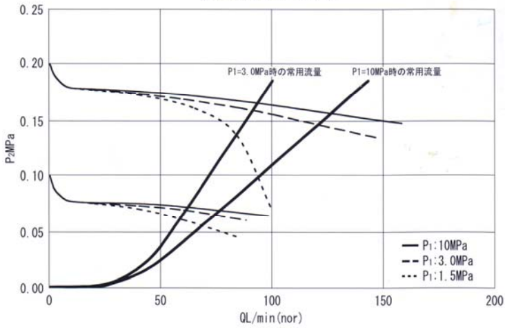
CMH-B503流量特性(N2ガス)
